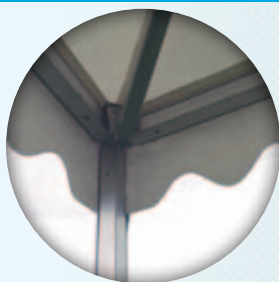
Accrochage des murs par lissage
