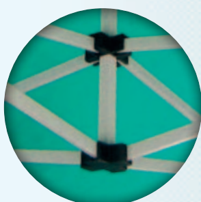
Pièces de connexions en nylon injecté (3 et 4 branches)
