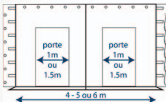
Mur porte double attaches élastiques et oeilletons
